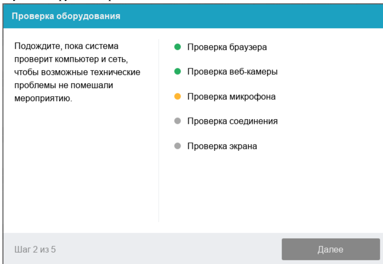
Рис. 7 — Проверка оборудования
