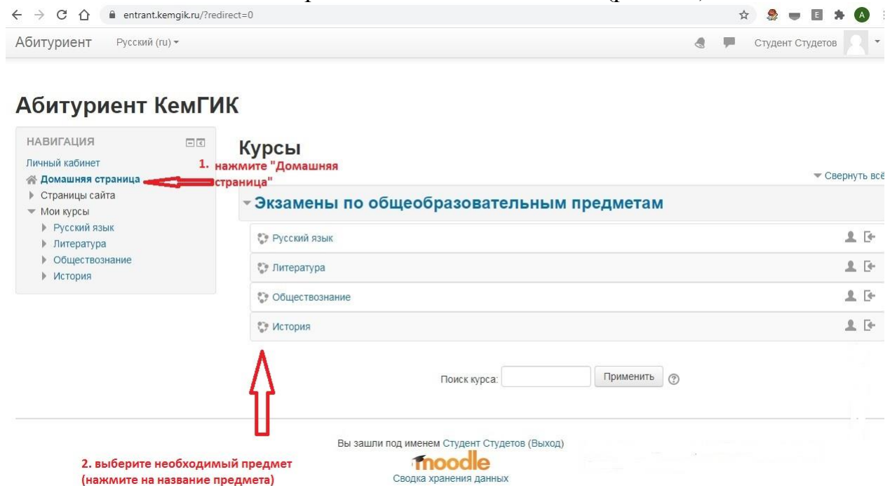
Рис. 4.1 - Домашняя страница
