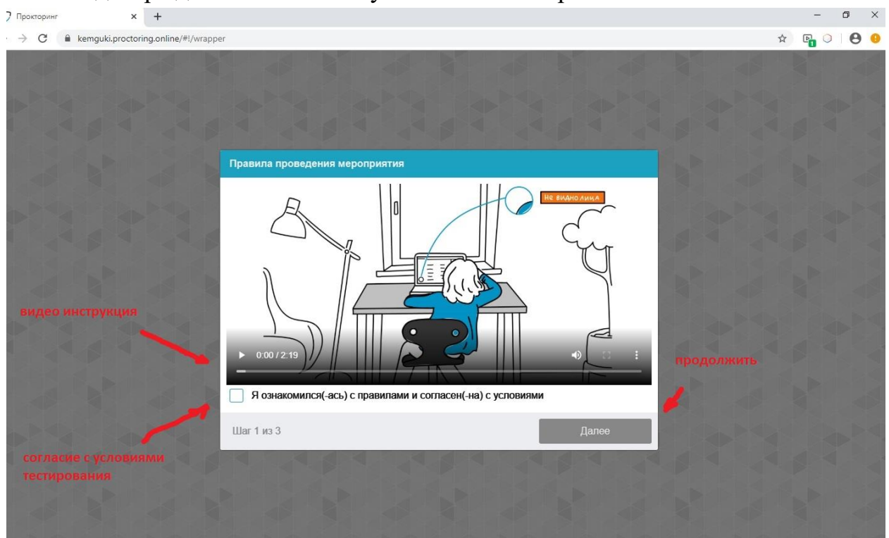
Рис. 6.2 - Начало тестирования
