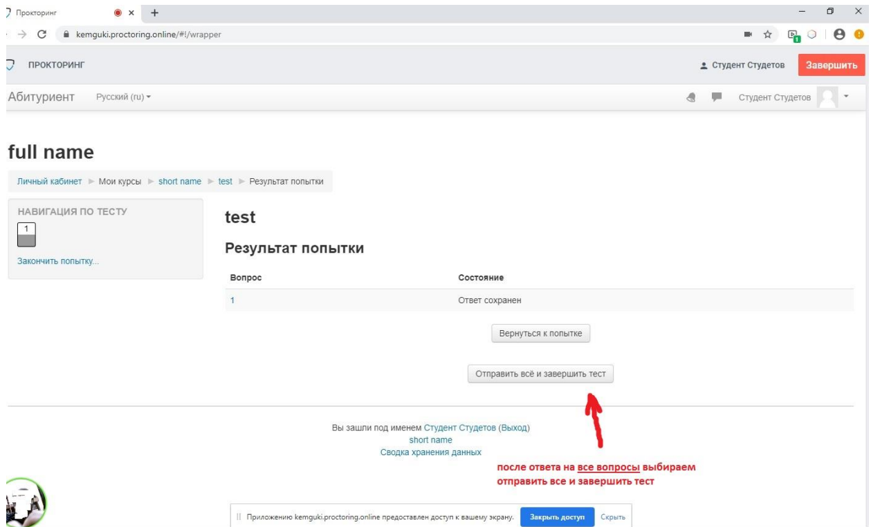
Рис. 12 - Завершение теста
