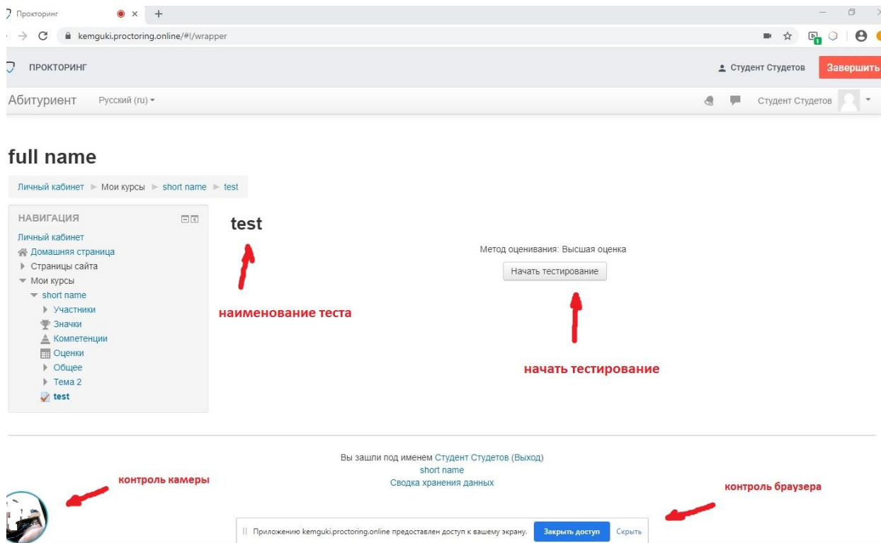
Рис. 10 - Начало тестирования
