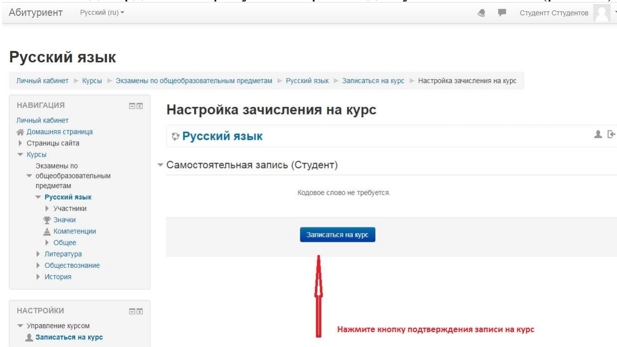
Рис. 4.3 - Подтверждение записи
